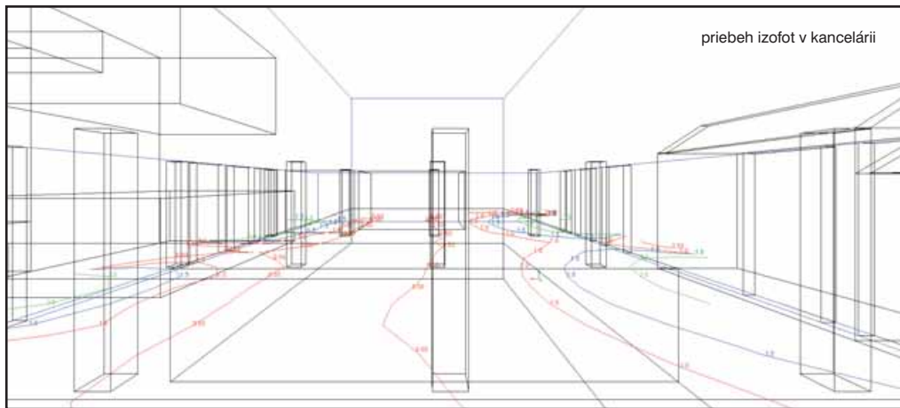
tienenie pomocou vertikálnych slnolamov – nevhodné riešenie
