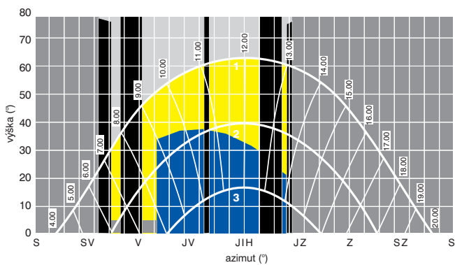
tienenie pomocou horizontálnych slnolamov – vhodné riešenie
